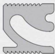
Zwischenprofil 4000 x 12,5 x 12 mm für Plattenstärken 16/19 mm
